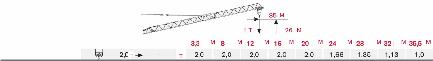
Максимальный вылет стрелы
