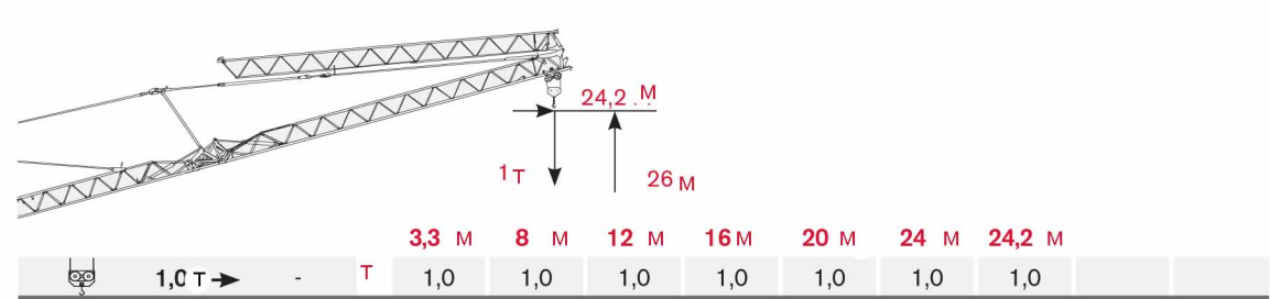
Сложенная и поднятая стрела 10°
