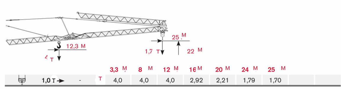
Сложенная и поднятая стрела
