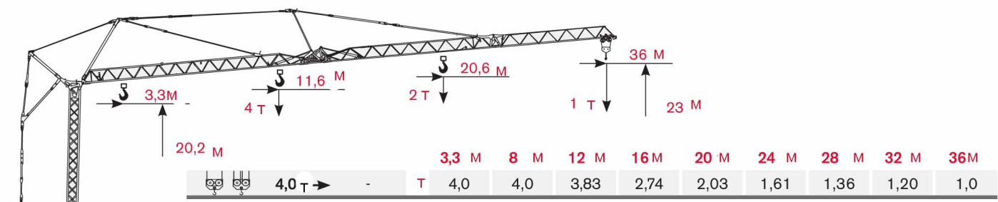
Сложенная и поднятая стрела 15°
