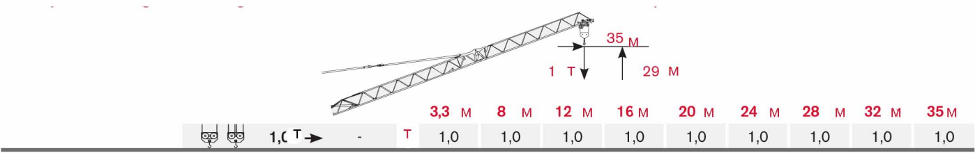
Сложенная и поднятая стрела 15°
