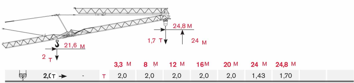
Сложенная и поднятая стрела
